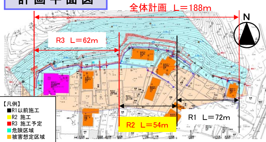
計画平面図
