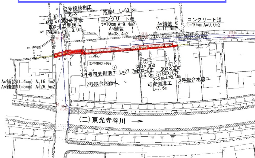
農業用水付替工 第2工区平面図
