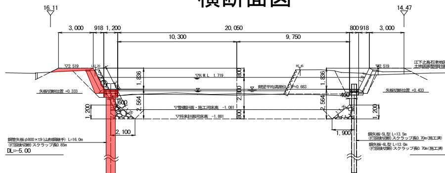
横断面図
